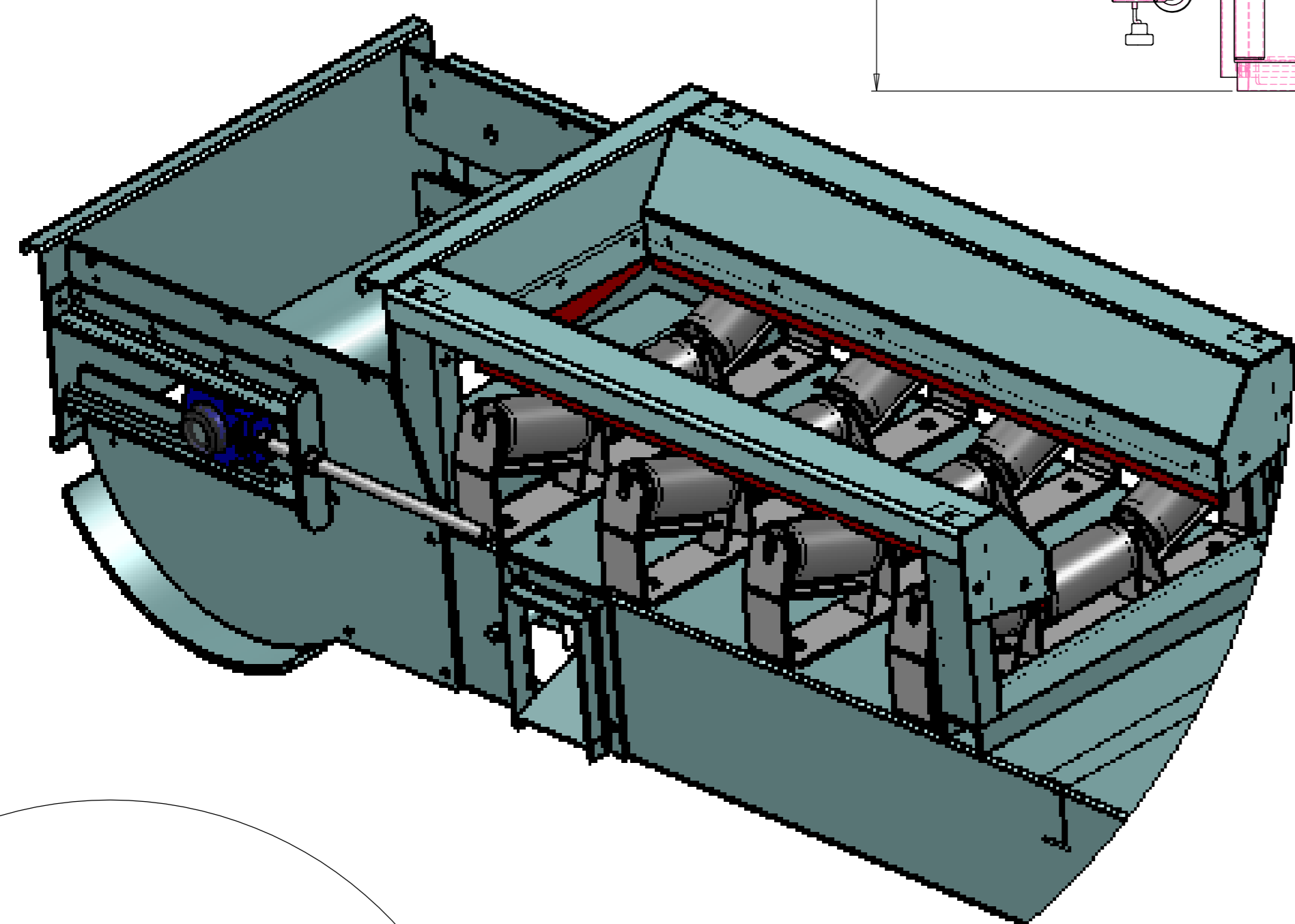
DÉTAIL D ECHELLE 2 : 15
